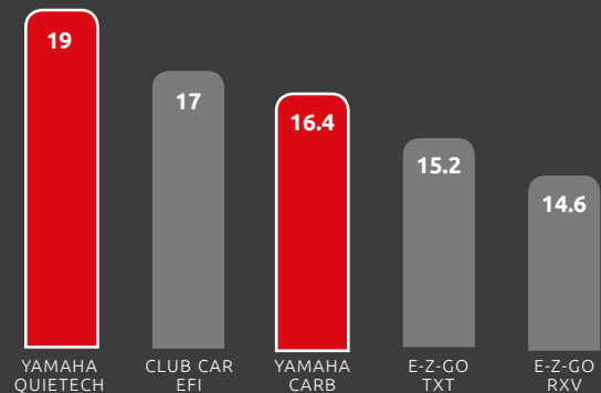
Yakıt Tüketimi (km/Litre)
