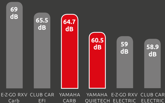
Quietech EFI. Ses Seviyesi
